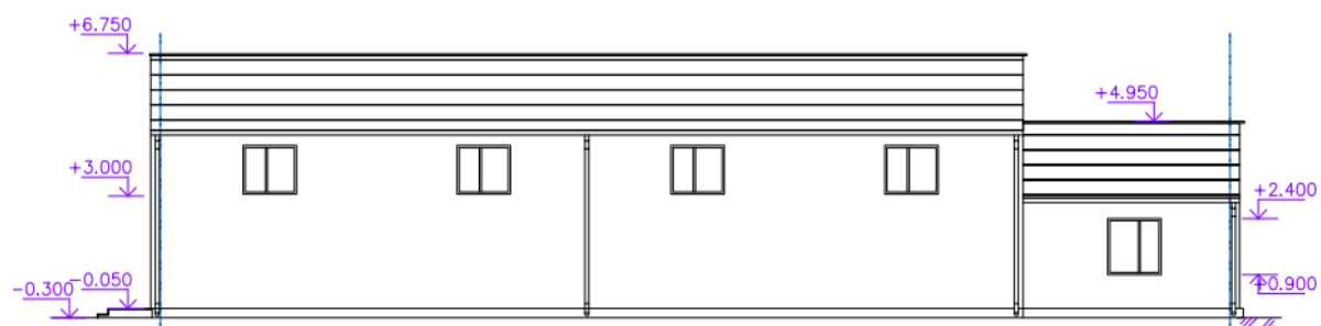
Гараж . Фасад в осях А-Б, Б-А
