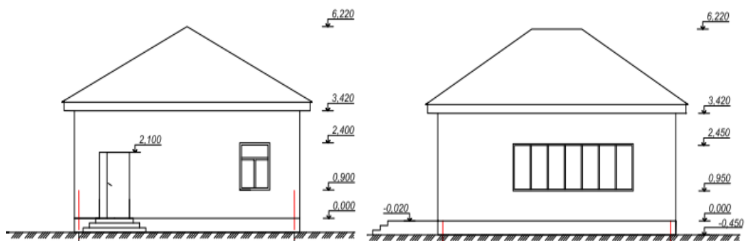
КПП. Фасад в осях А-В, 1-2
