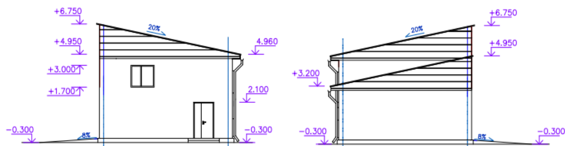
КПП. Фасад в осях В-А, 2-1
