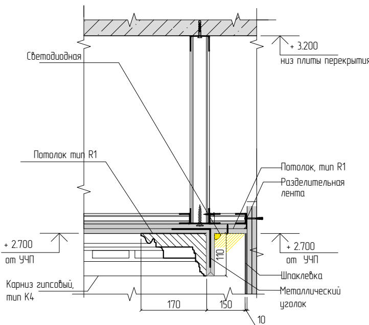
Разрез 2-2 Устройство закарнизной подсветки в пом. N 4 (санузел).
