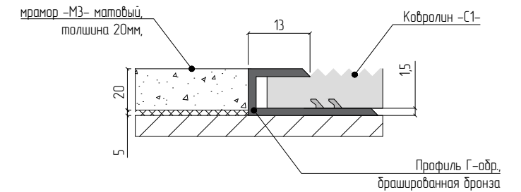
Деталь облицовки портала и порожек пом. N4 (су) Разрез 7-7
