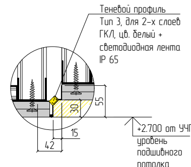
Узел 8 Устройство закарнизной подсветки в пом. N 5 (душевая).
