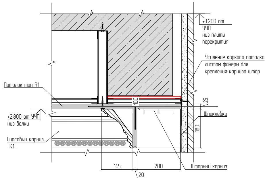
Разрез 1-1 Устройство шторной ниши и примыкания к балке двухсоставного гипсового карниза
