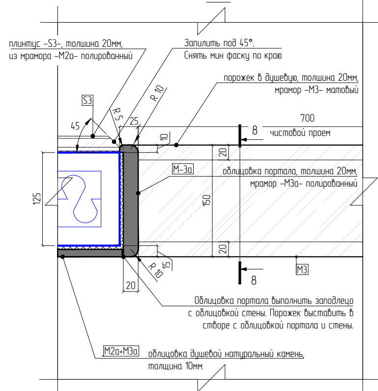
Деталь облицовки портала и порожек пом. N5 (душевая) ПЛАН
