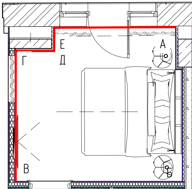
План с маркировкой разверток
