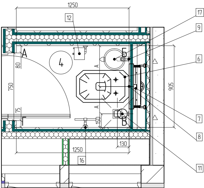
План с привязкой сантехники и маркировкой оборудования.
