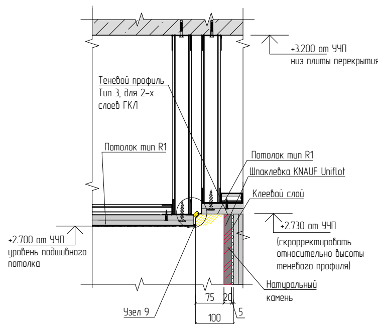
Разрез 8-8 пом. 2 (гардеробная)
