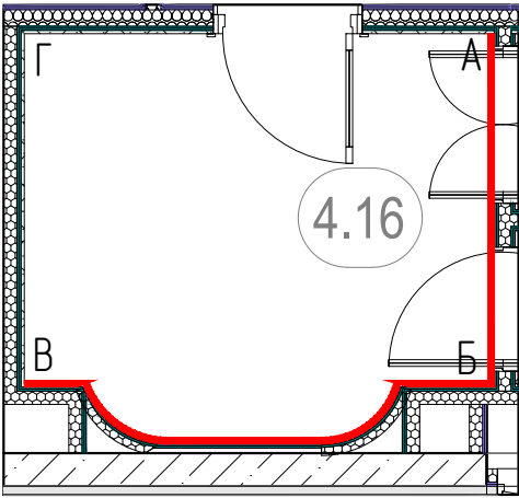
План с маркировкой разверток. М 1:50
