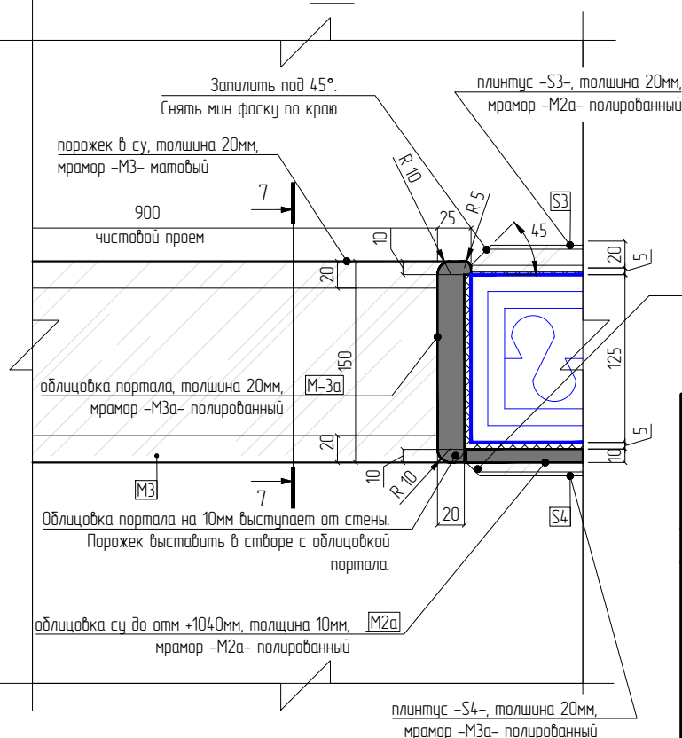
Деталь облицовки портала и порожек пом. N4 (су) ПЛАН
