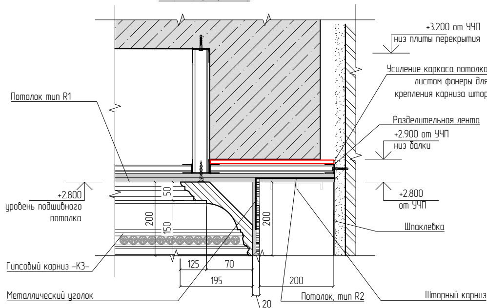
Разрез 8-8 пом. 2 (гардеробная)
