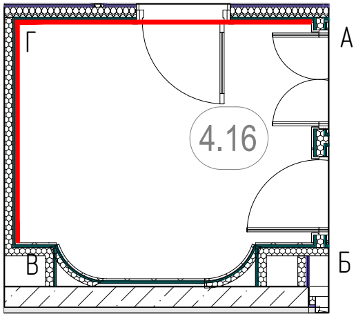
План с маркировкой разверток. М 1:50
