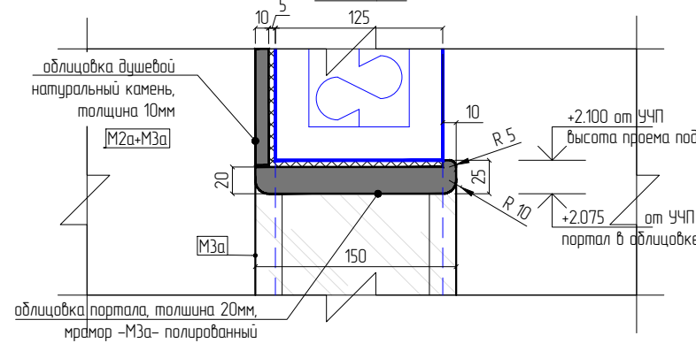
Деталь облицовки верха портала пом. N5 (душевая) Разрез 8-8
