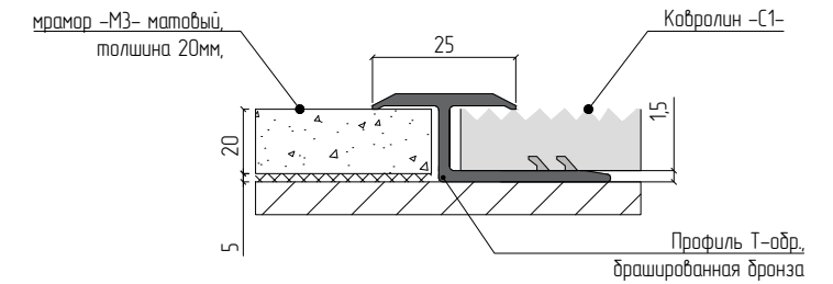
Стык напольного покрытия. Вар. профиль 2
