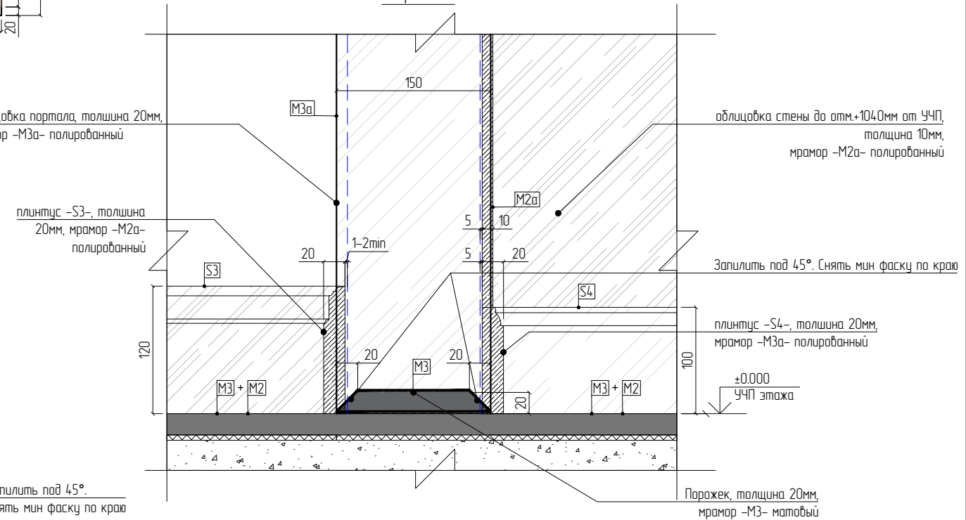
Деталь облицовки портала и порожек пом. N4 (су) Разрез 7-7
