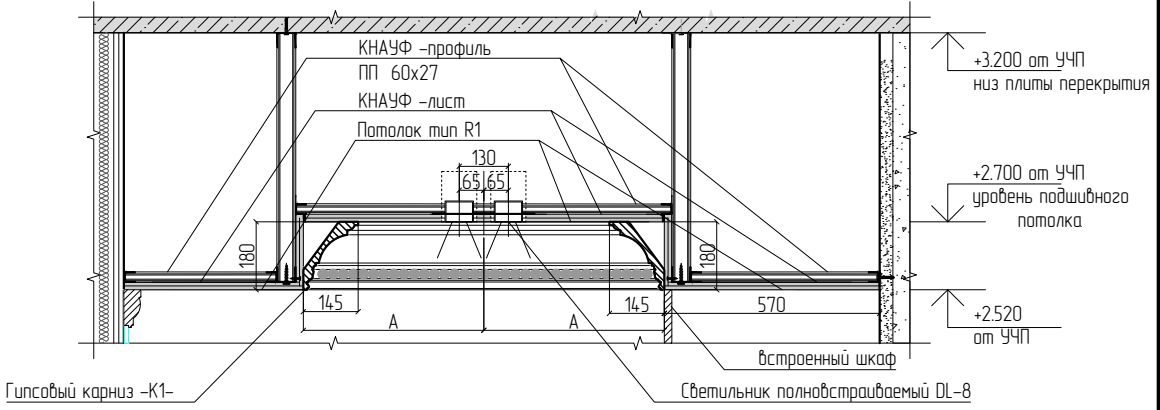
Разрез 6-6 пом. 2 (гардеробная)
