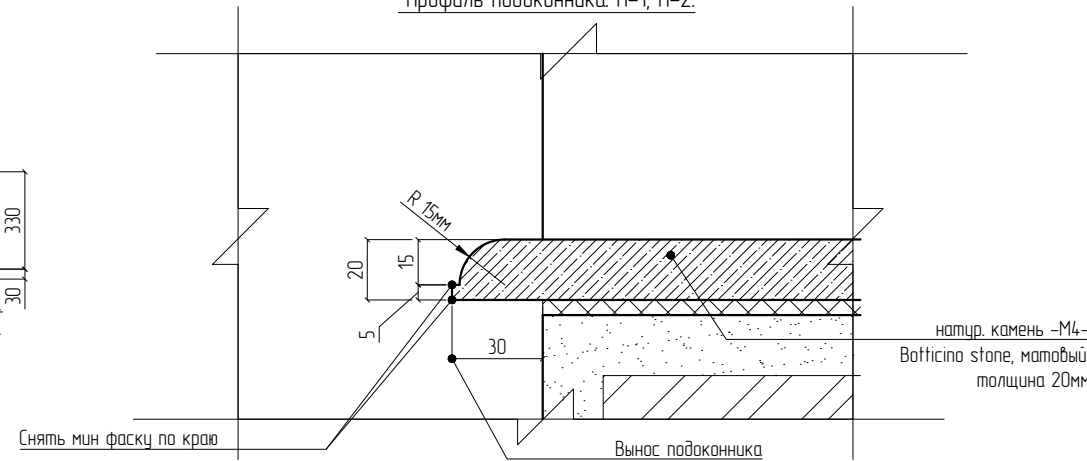
Деталь к узлу 4. Профиль подоконника. П-1, П-2.
