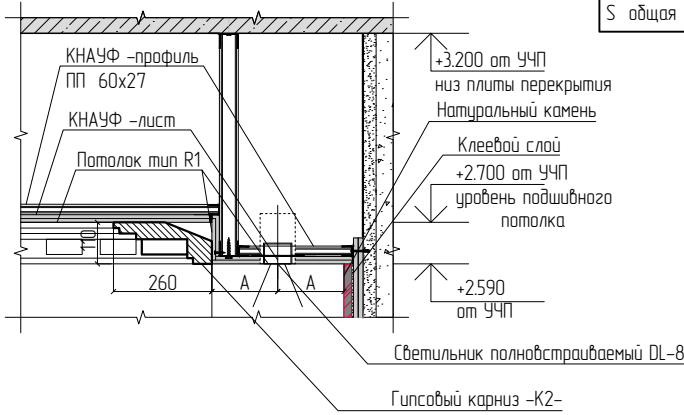
Разрез 6-6 пом. 2 (гардеробная)
