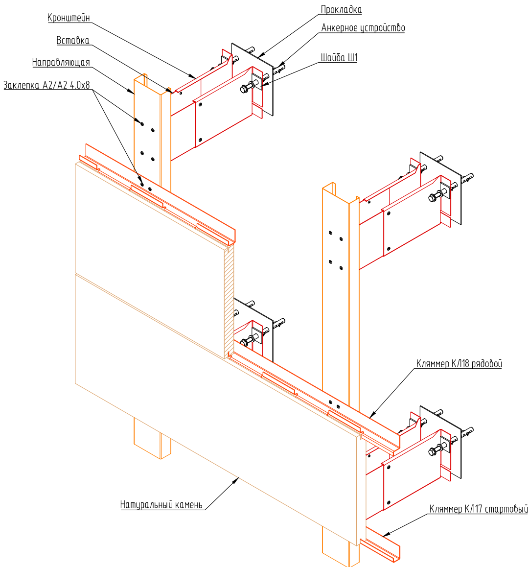
Аксонетрическая схема
