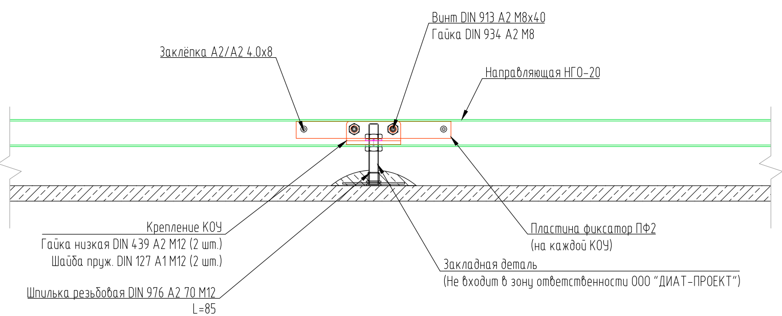
Вид А
