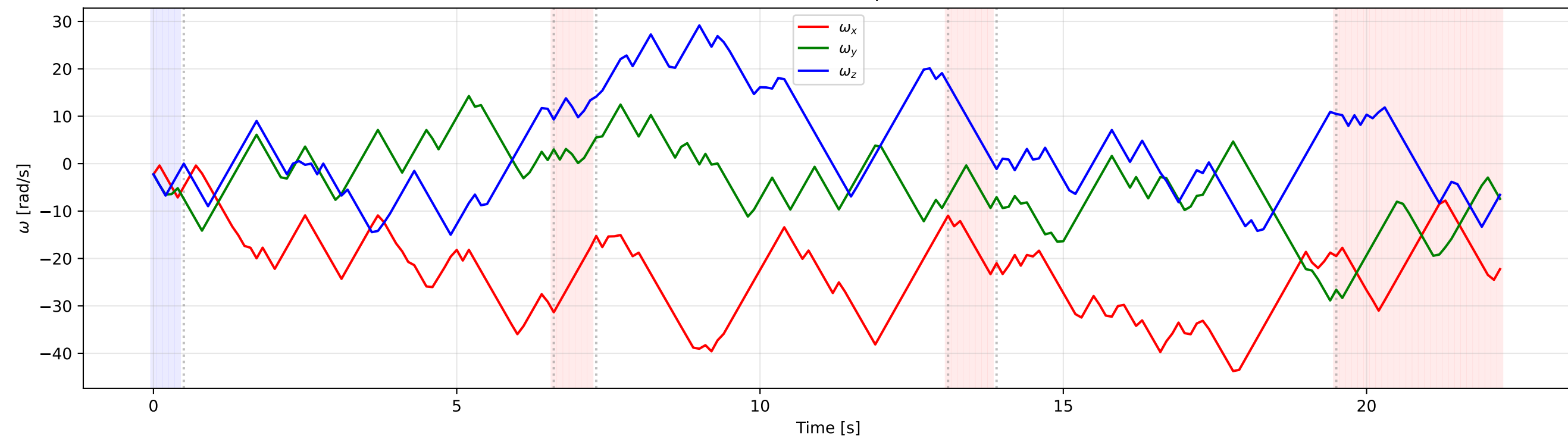
(d) Reaction wheel speeds \omega(t)
