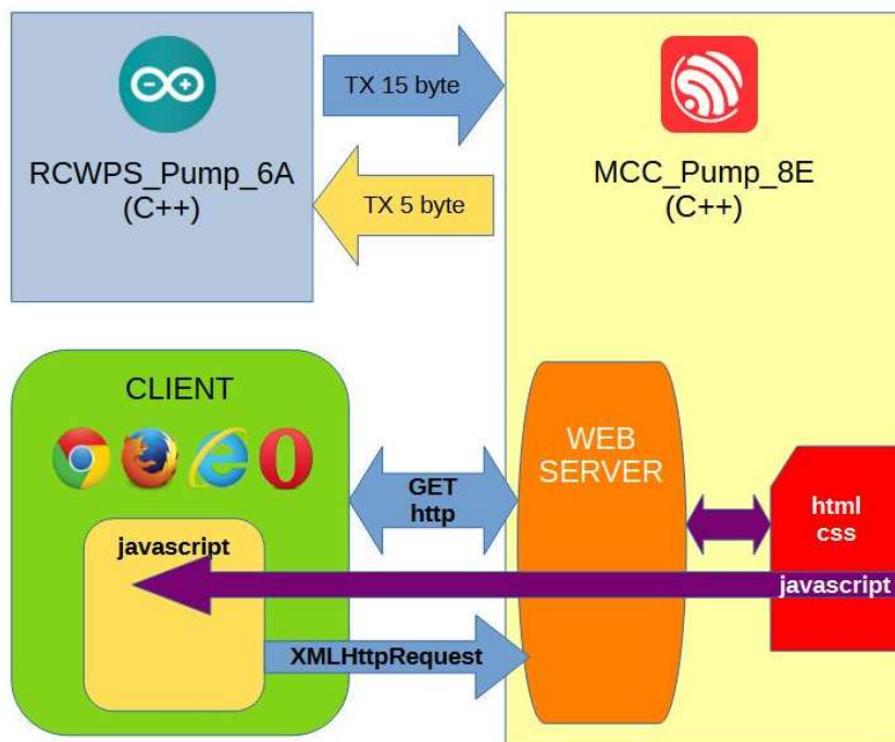
Рисунок 21 – Структурная схема информационного обмена
