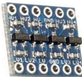
Рисунок 17 – Модуль преобразователь уровней 5В – 3,3В 4х канальный
