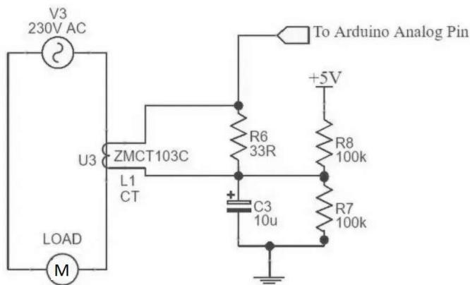
Рисунок 8 – Схема сопряжения трансформатора тока со входом контроллера
