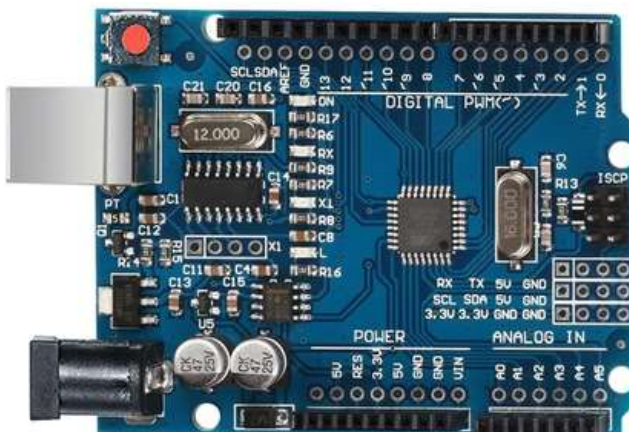
Рисунок 3 – Плата контроллера Arduino UNO
