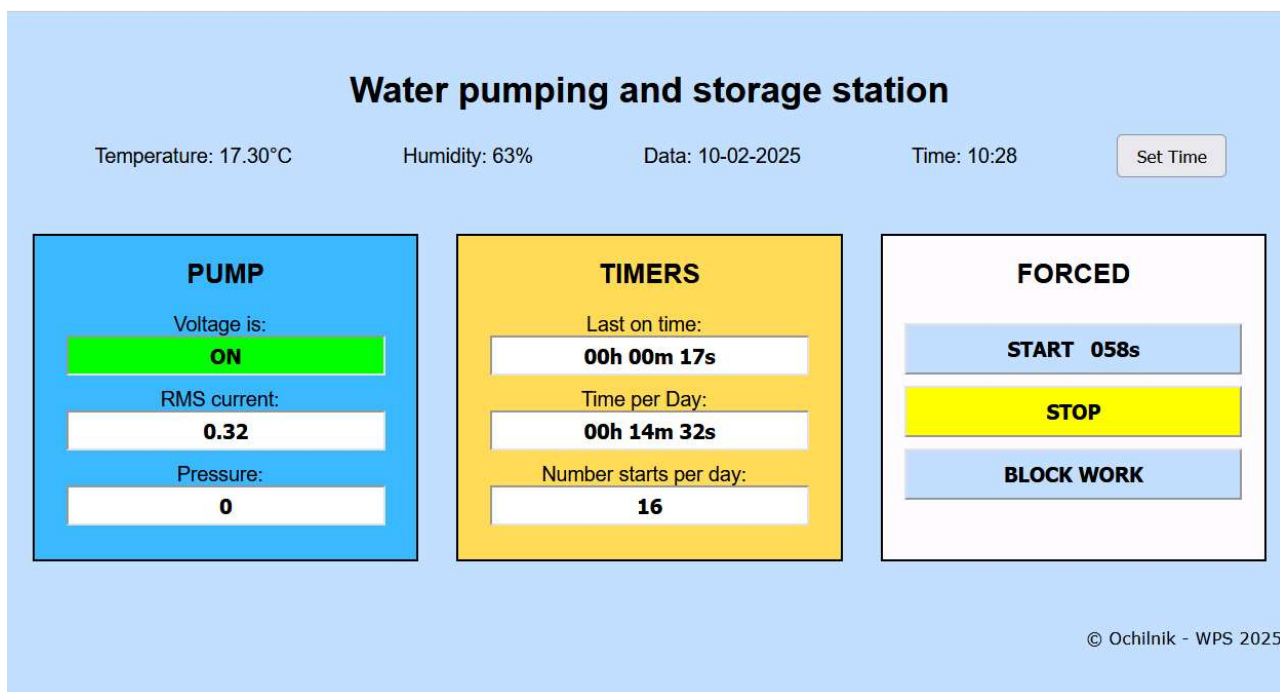
Рисунок 26 – Веб-интерфейс системы контроля НАС
