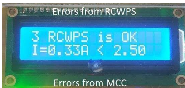
Рисунок 24 – Назначение индикации экрана 3 дисплея MCC
