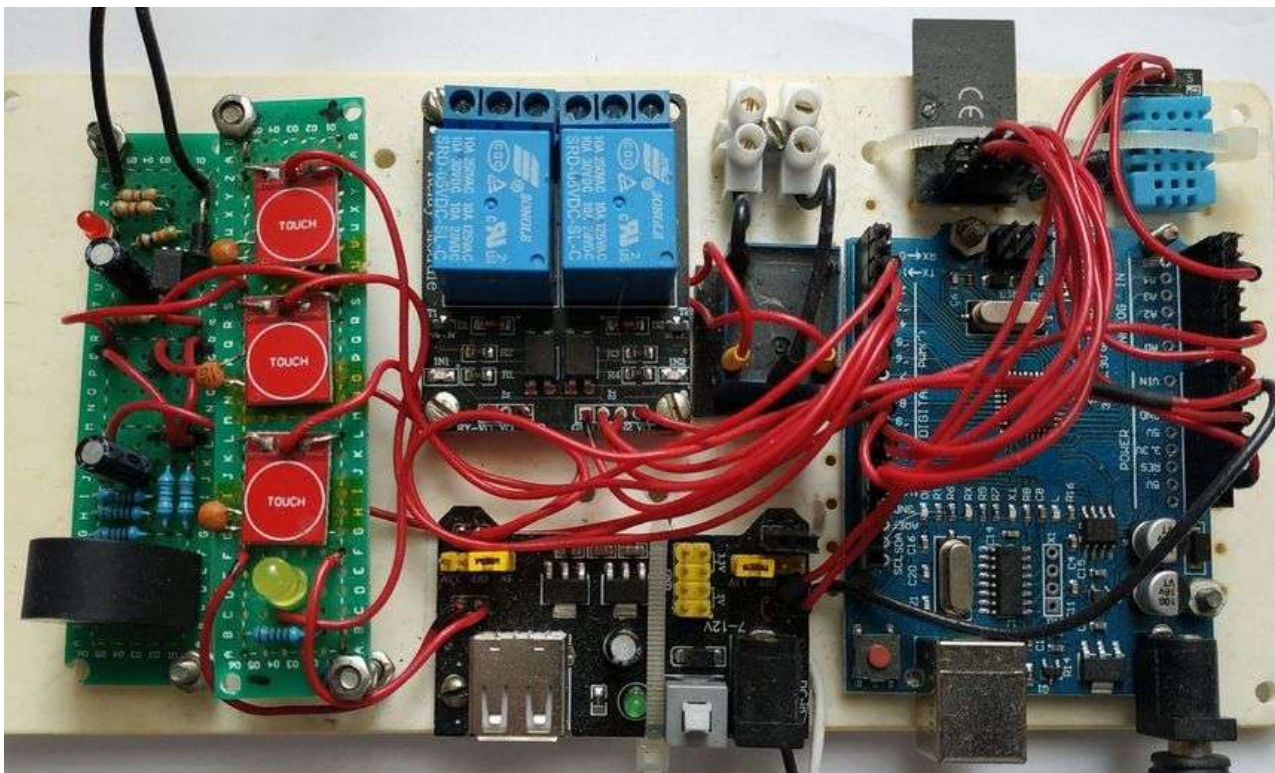
Рисунок 11 – Контроллер RCWPS
