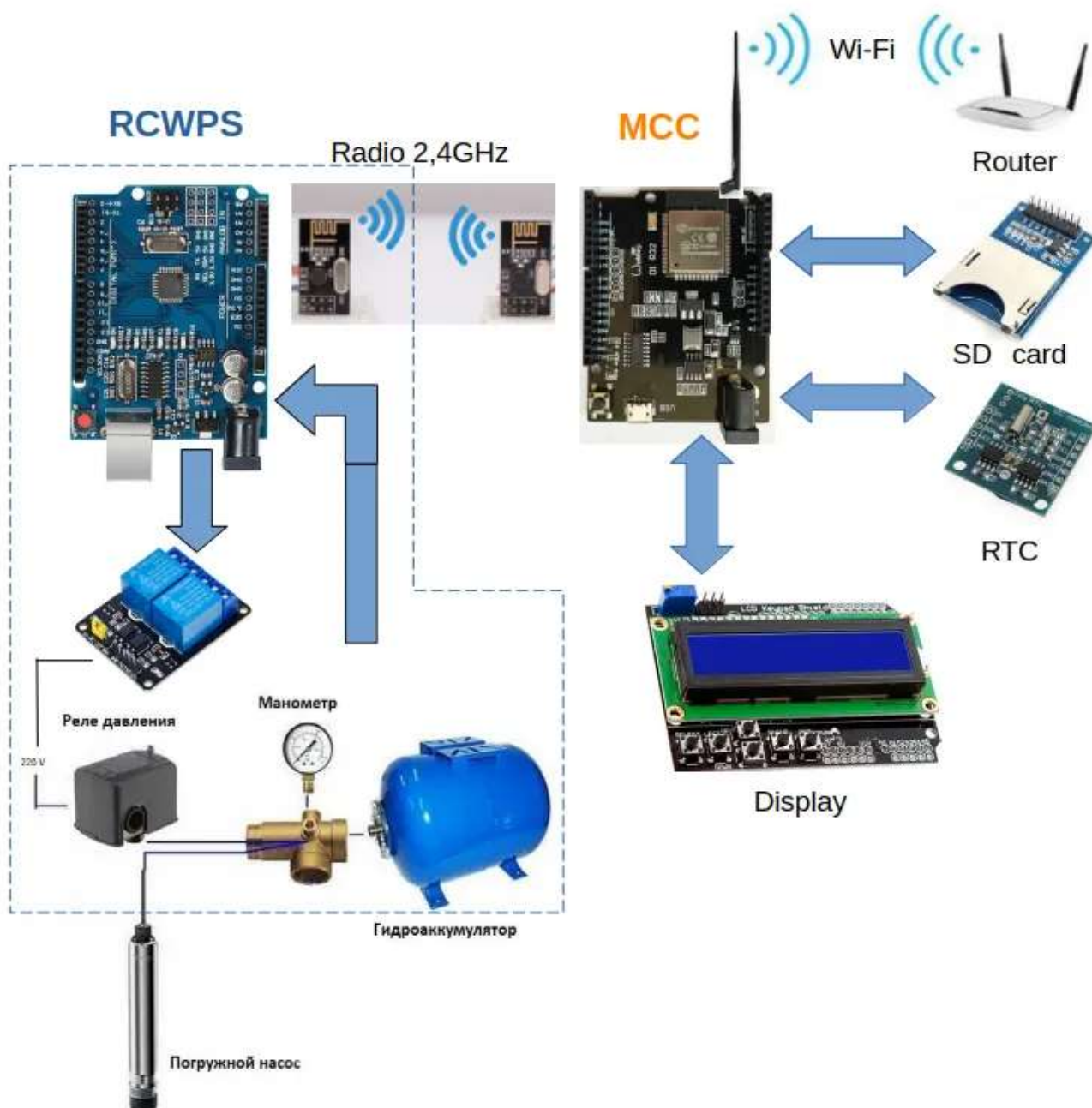
Рисунок 1 — Структурная схема системы контроля НАС подачи воды
