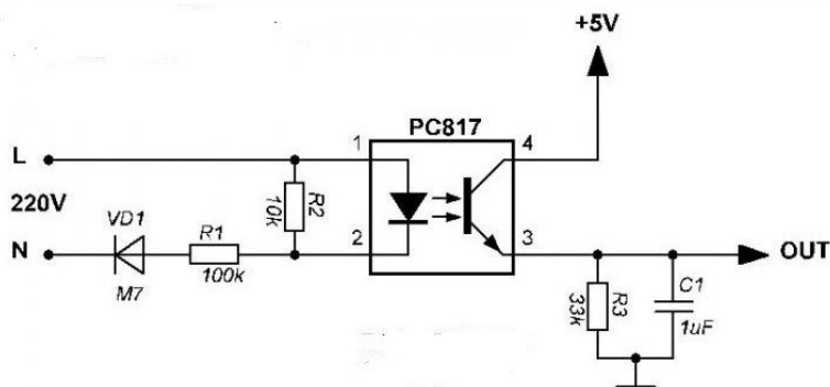
Рисунок 7 – Схема сопряжения цепи AC220В со входом контроллера
