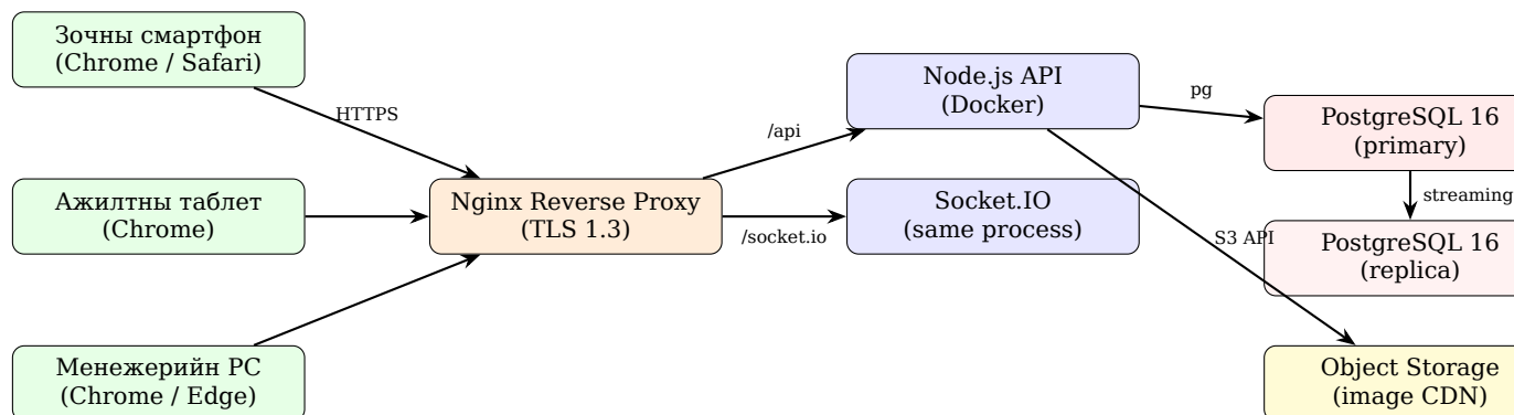
Figure 3.3: Системийн хэрэгжүүлэлтийн (deployment) диаграм
