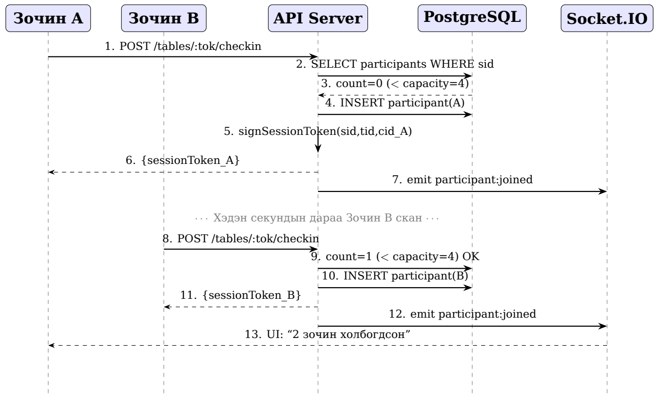
Figure 3.18: Олон төхөөрөмжийн check-in дарааллын диаграм
