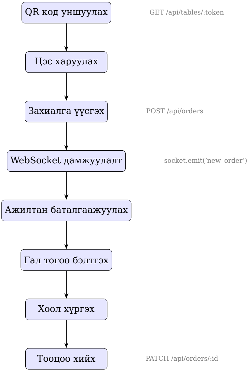
Figure 2.1: Системийн ерөнхий үйл ажиллагааны урсгал
