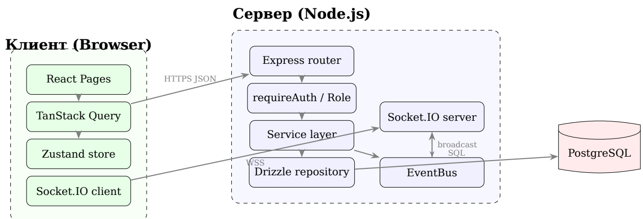
Figure 3.2: Системийн компонент диаграм
