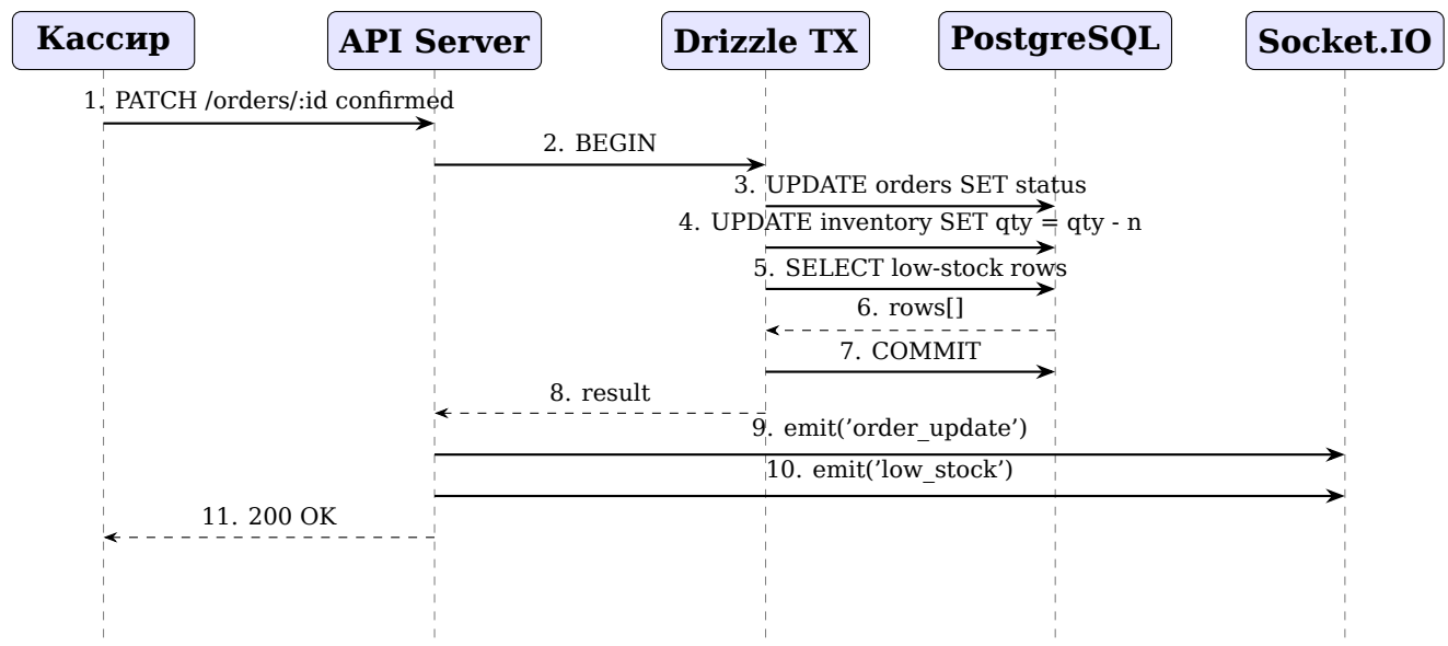
Figure 3.8: Нөөцийн автомат хасалт ба low-stock мэдэгдлийн дараалал
