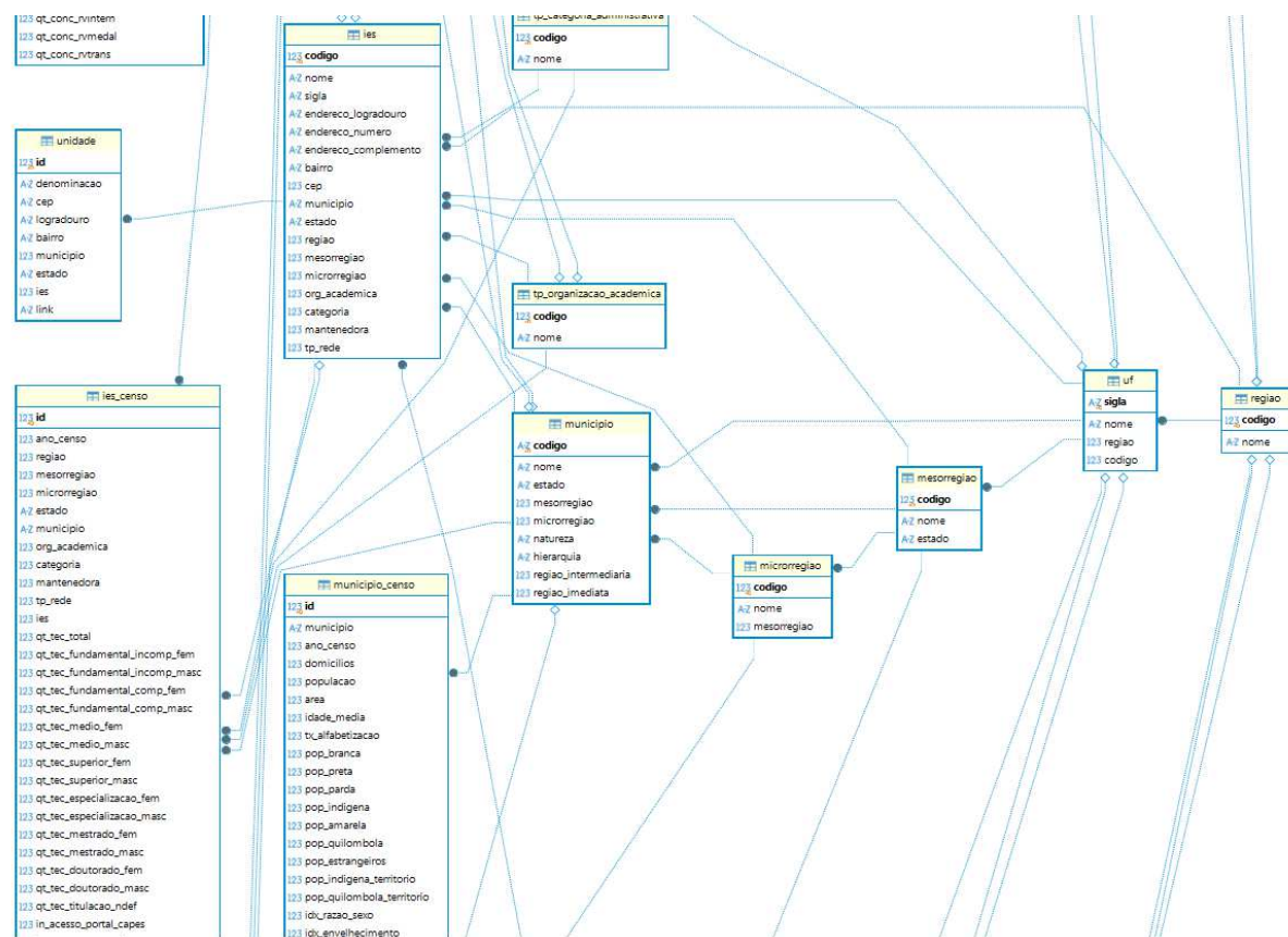
Figura 18 - Parte do modelo de dicionário de dados do Data Warehouse projetado
