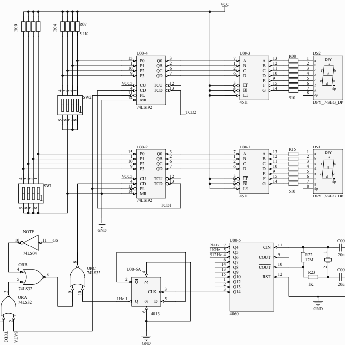
PART-00-可预置时间倒计时电路原理R00-49
