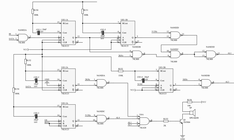
PART-03-各种警告音电路R150-199
