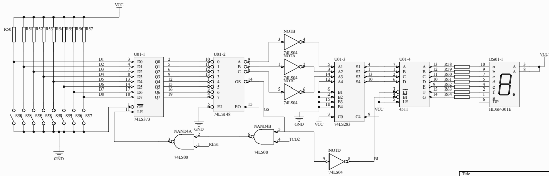
PART-01-抢答输入、锁存、显示电路R50-99
