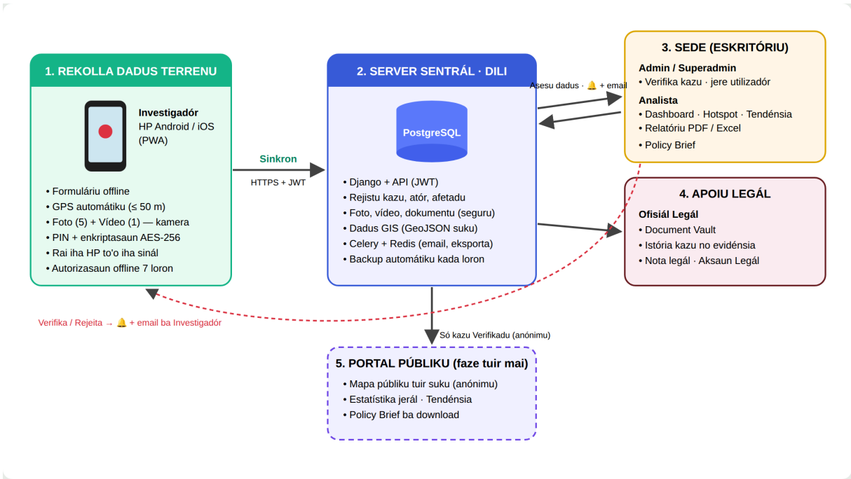
Figura 1. Arkitetura SMKRE — husi terrenu to'o sede no portal públiku
