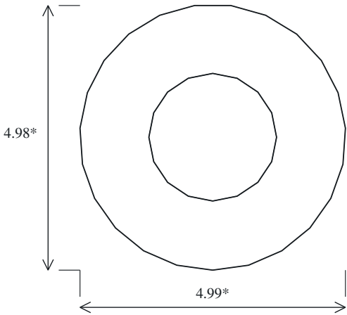
Вид по -X · Y/Z · М 10:1
