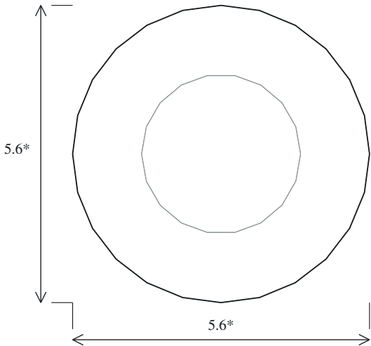
Вид по −Z · X/Y · М 10:1
