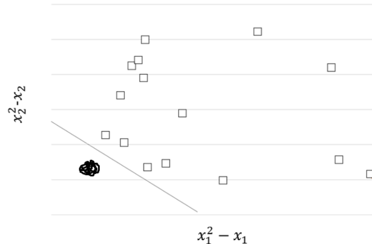
(b) 变换后空间的决策边界
