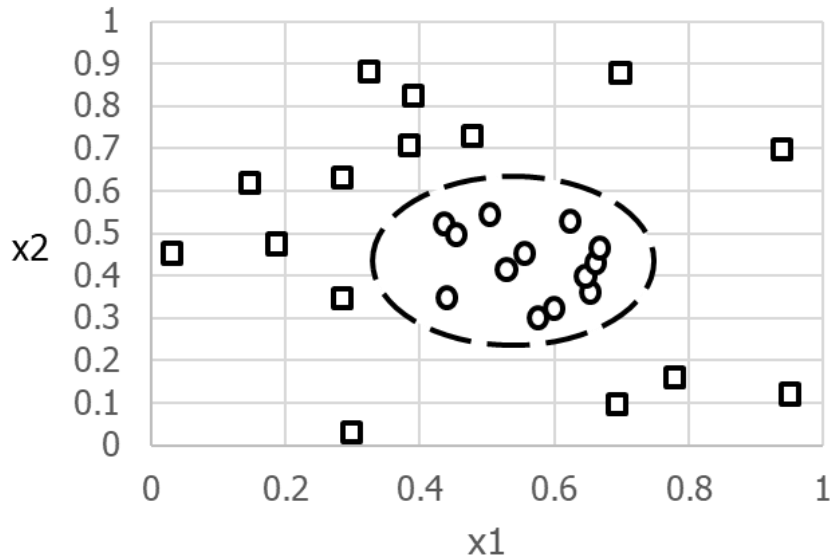
原二维空间中的决策边界
