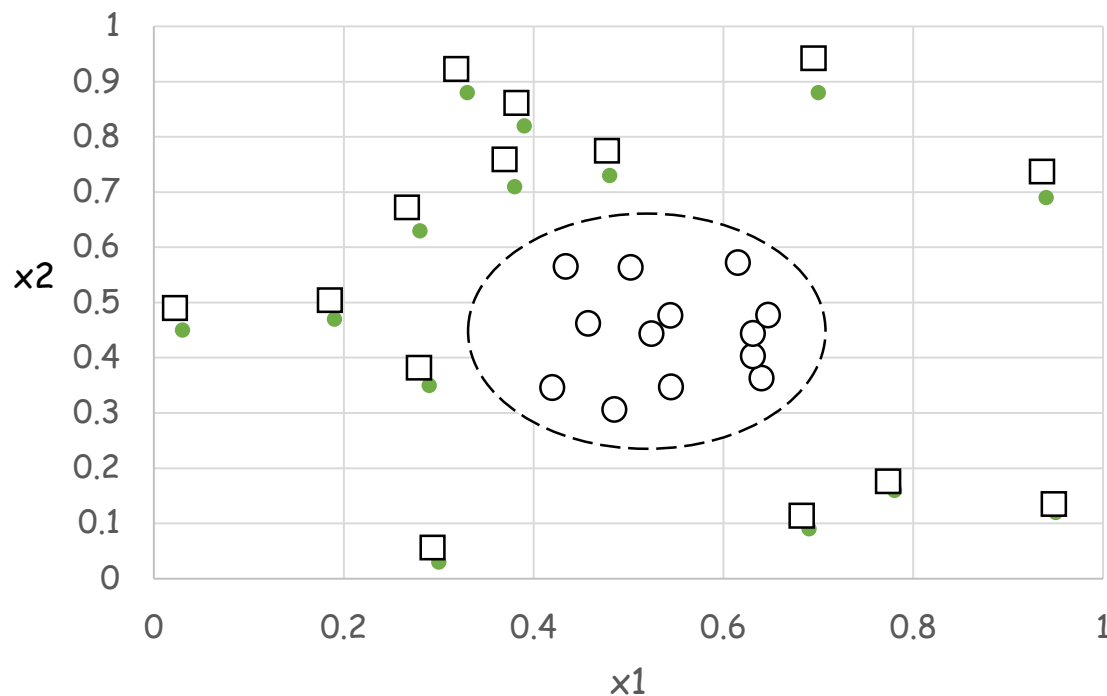
原二维空间中的决策边界
