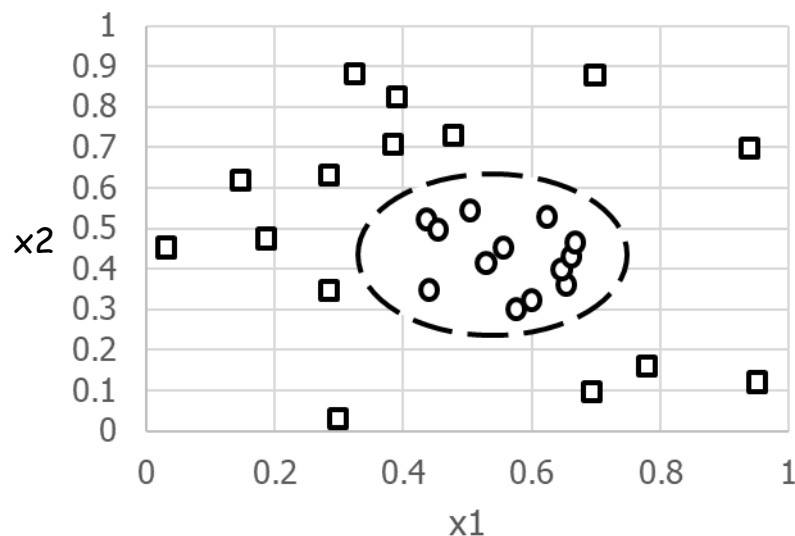
(a) 原二维空间中的决策边界
