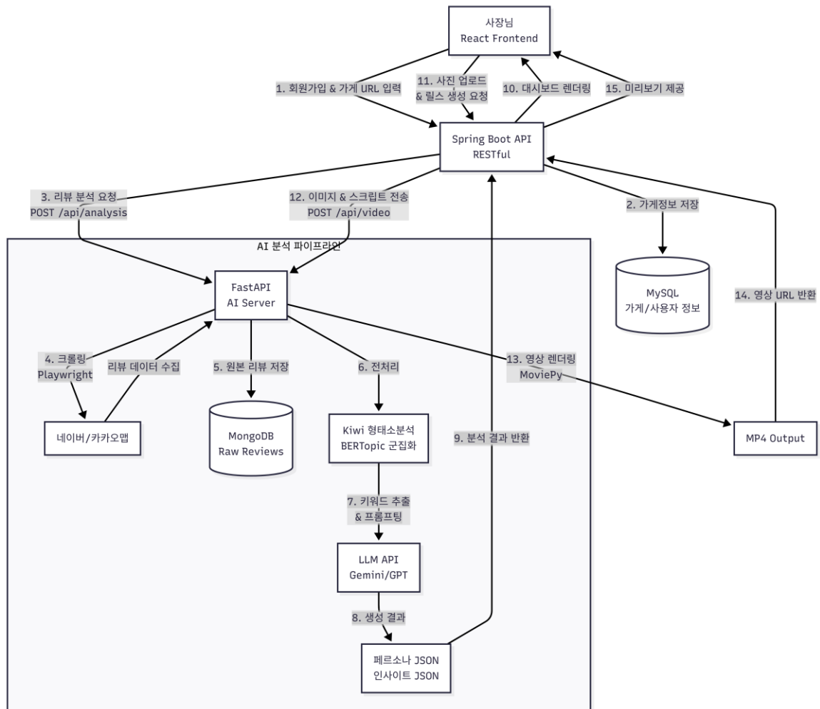
PULSE 통합 기술 아키텍처
