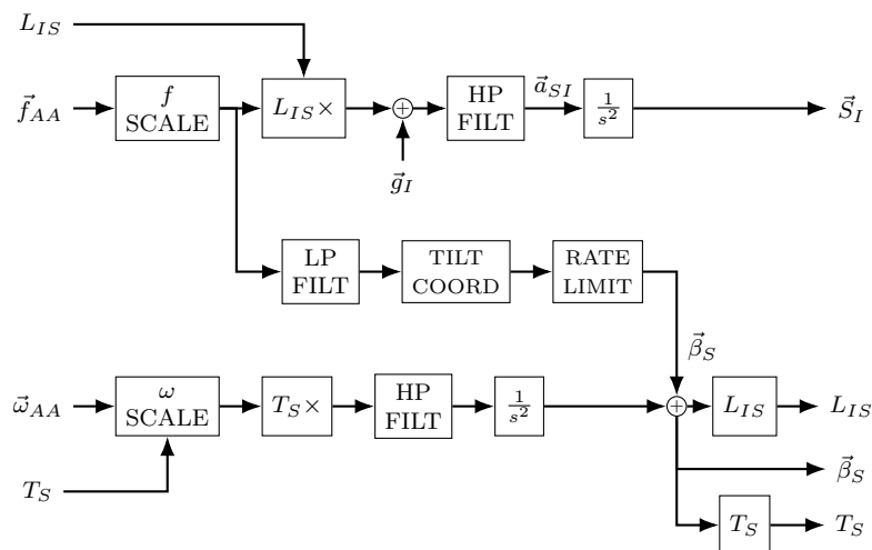
Figura 1: Representación del Classical Washout, de Nahon y Reid.
