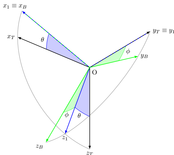
Figura 4: Diagrama de la rotación mediante ángulos de Euler
