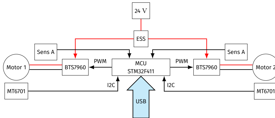
Figura 2: Funcionamiento general del sistema de control de movimiento
