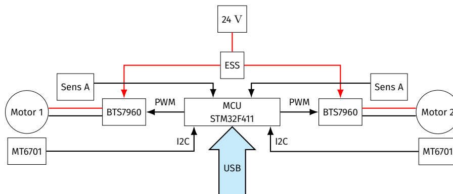
Figura 1: Funcionamiento general del sistema de control de movimiento
