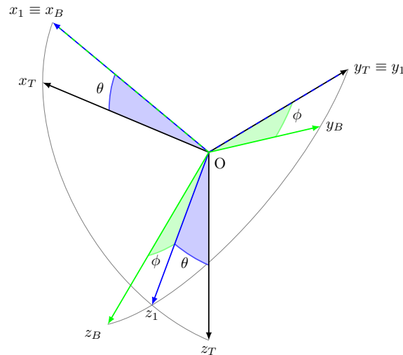
Figura 3: Diagrama de la rotación mediante ángulos de Euler
