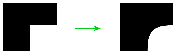
Figura 3.1: Ejemplo de cómo un redondeo permite la impresión de un voladizo
