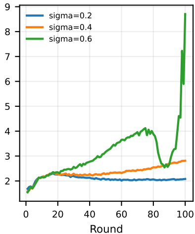
Base gradient norm
