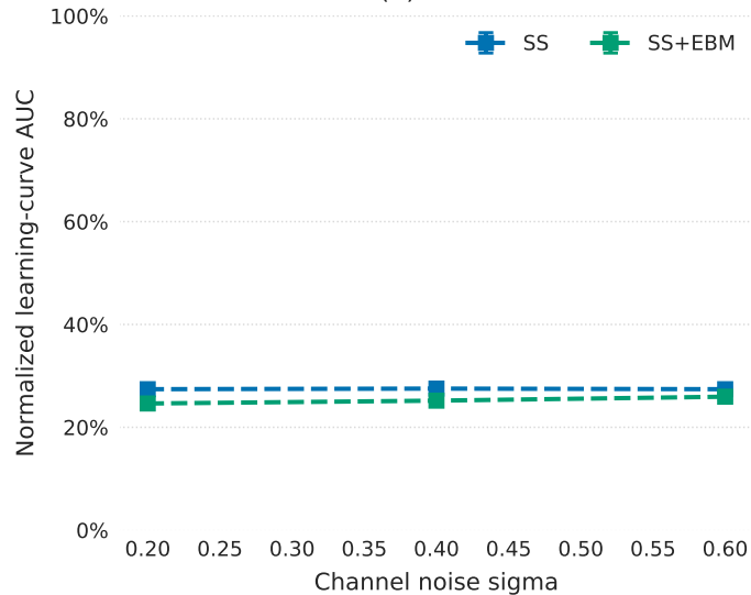
(b) CART
