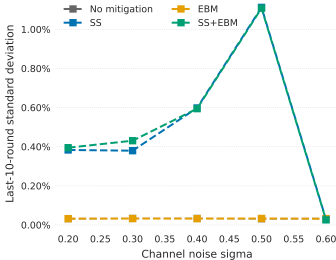
(b) CART
