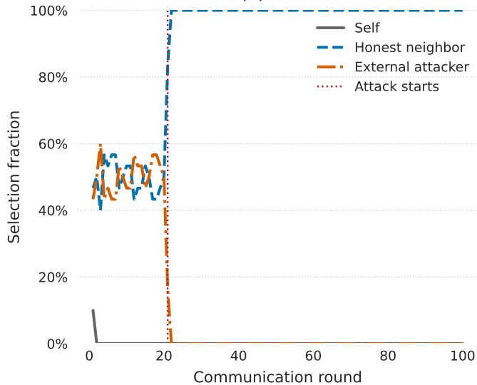
(b) CART
