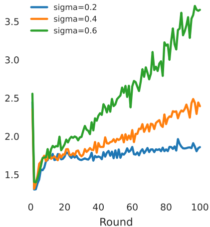
Base gradient norm
