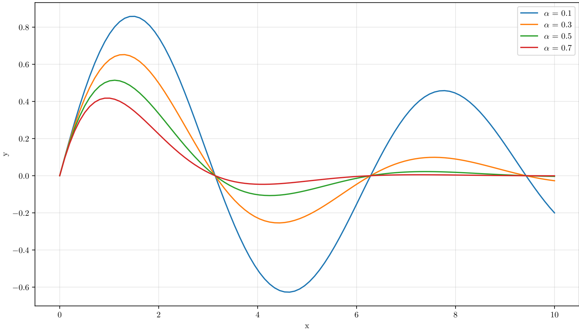
Parameter Sensitivity
