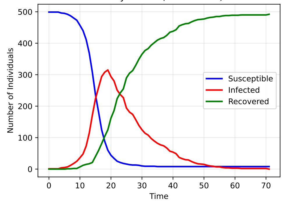
SIR Dynamics (ER Network)
