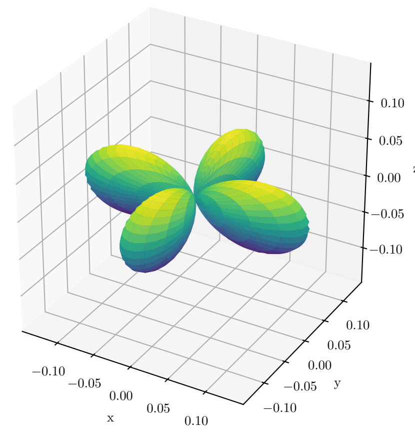
3d x^2-y^2 : \text{Re}(Y_2^2)
