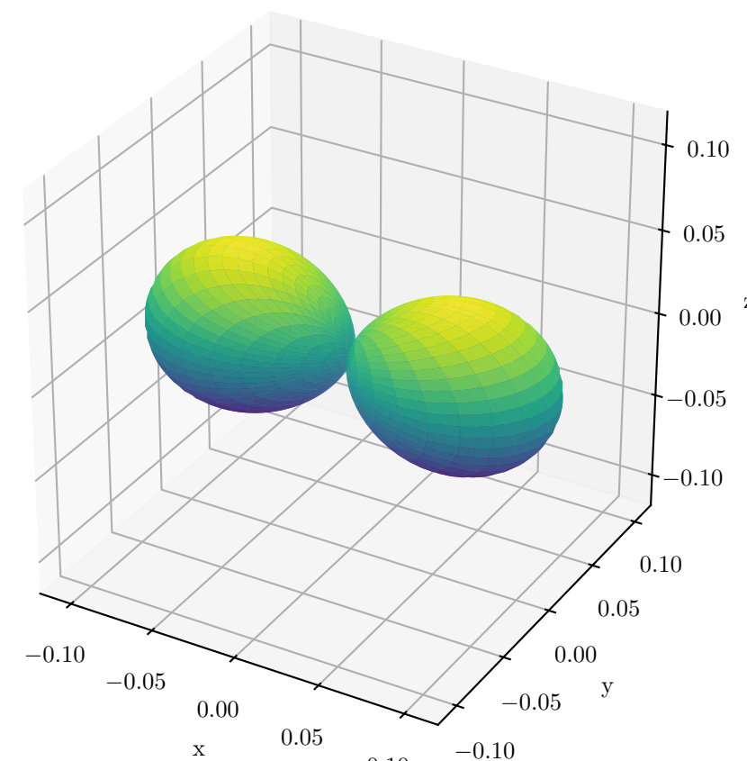
3d x^2-y^2 : \text{Re}(Y_2^2)
