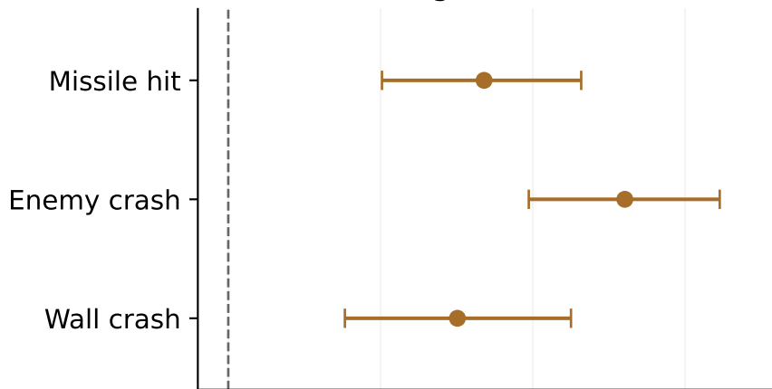
Gambling · 200-350 ms
