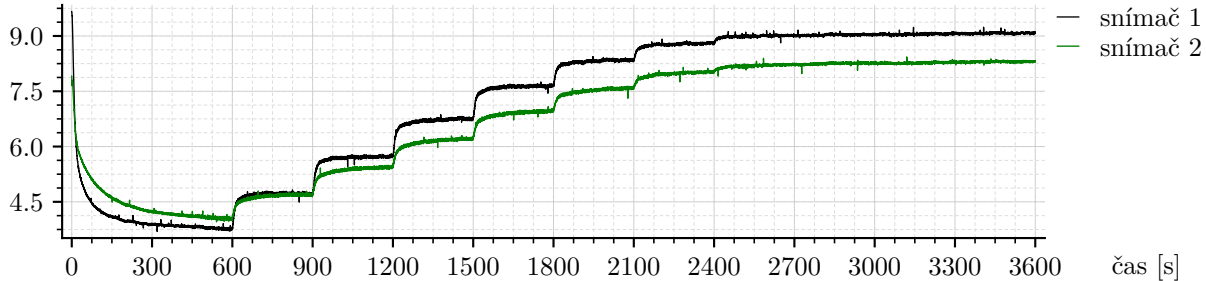
[V] Výstupné signály (snímač 1 a snímač 2)
