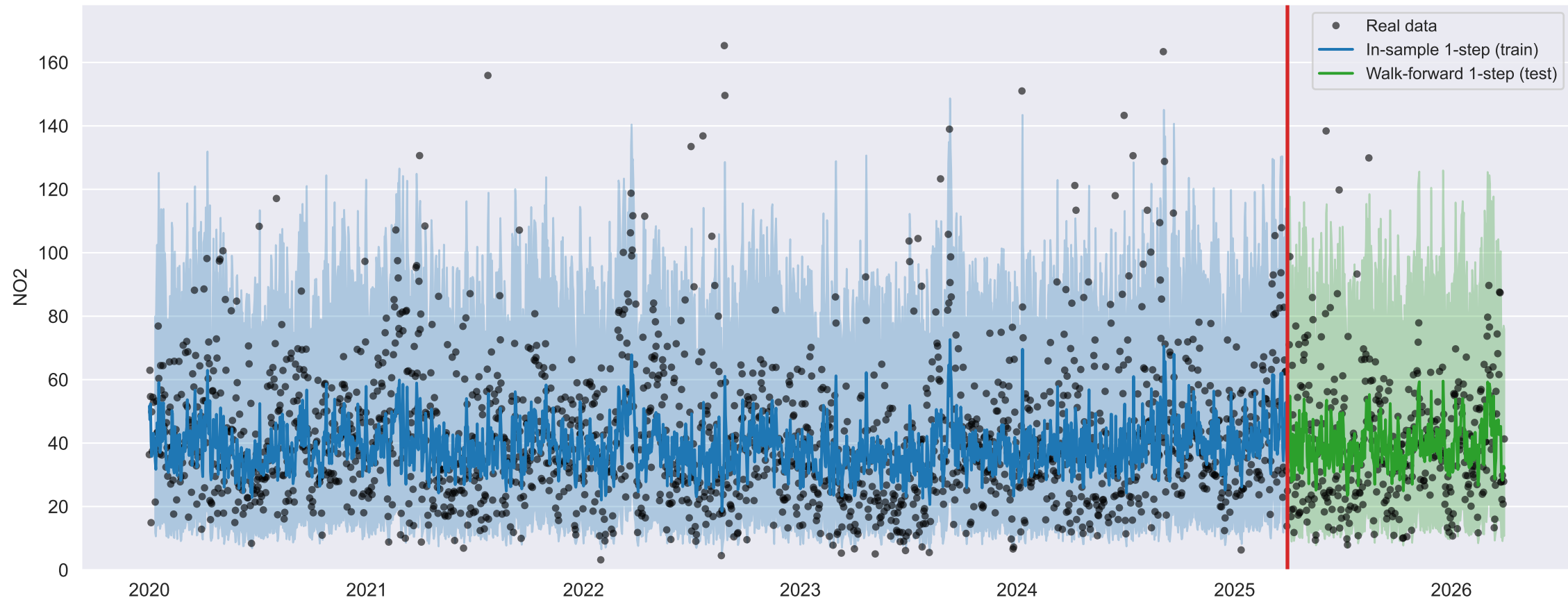
VARX (dummies + meteo) — NO2
