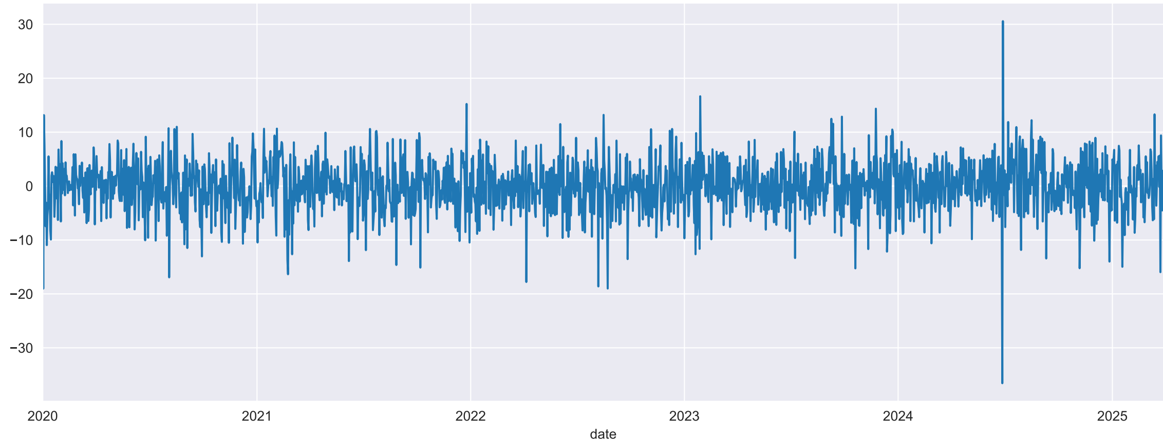
O3 - residuals
