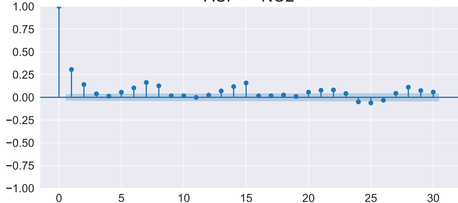
ACF — NO2
