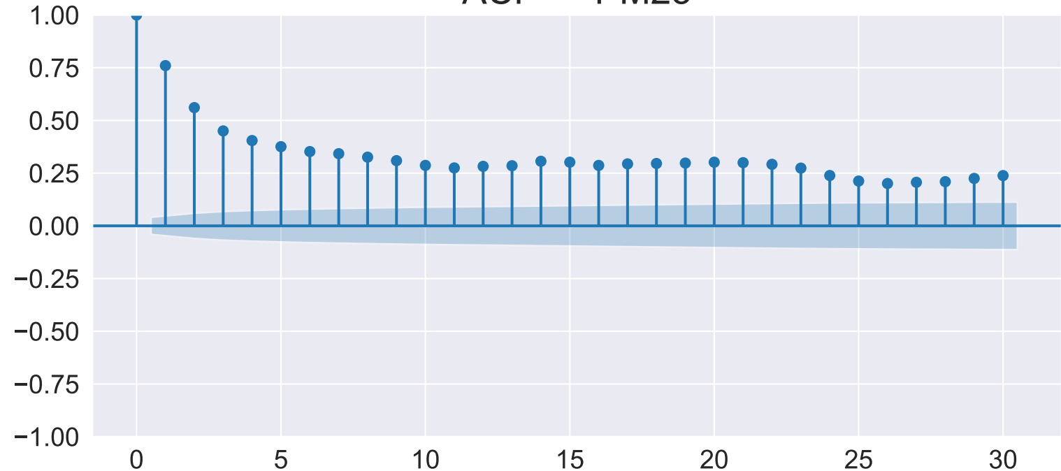
ACF — PM25
