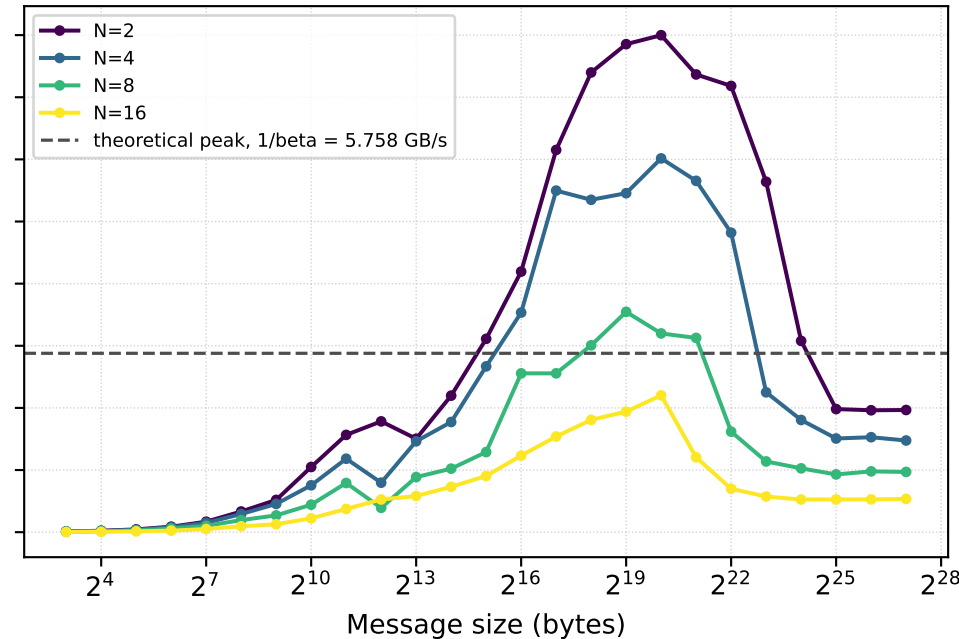
MPI_Allreduce, default
