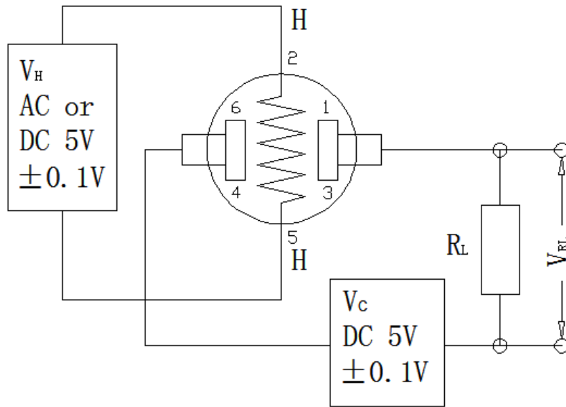
图 2： MQ-3B 测试电路
