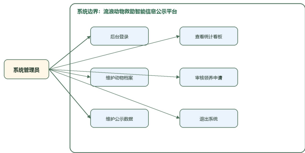
系统管理员用例图
