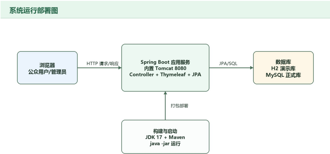
图 4-1 系统总体架构图
