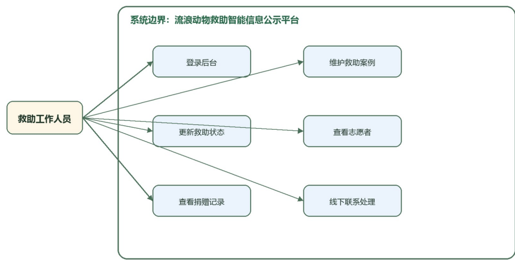
救助工作人员用例图
