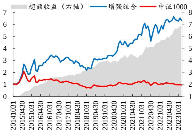
图20: TRCF 在中证 1000 中超额收益稳定
