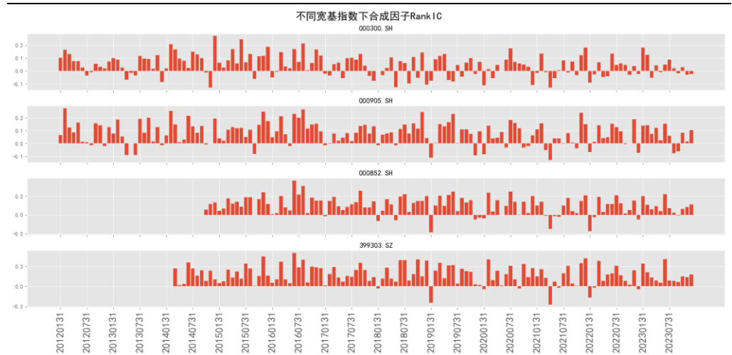
图16：不同宽基指数下 TRCF 的时序 RankIC
