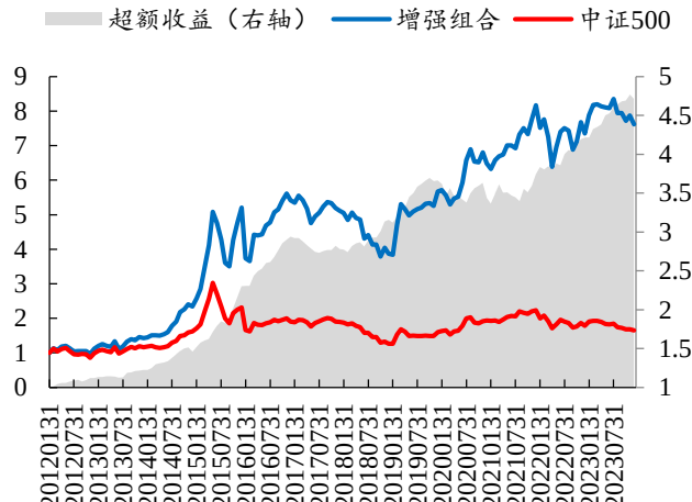
图19: TRCF 在中证 500 中超额收益波动较大
