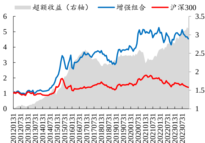
图18: TRCF 在沪深 300 中偶尔出现失效风险
