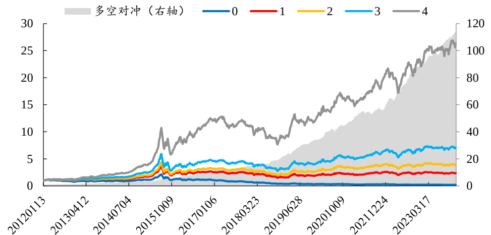
图23：周频调仓下换手率收敛因子多头收益提升明显
