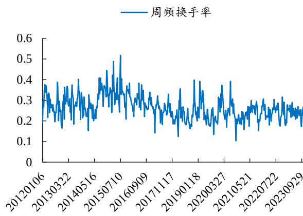
图26：周频调仓时 TRCF 周均换手率约 26%
