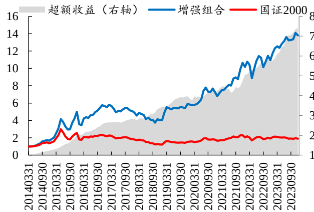
图21: TRCF 在国证 2000 中增强表现最优
