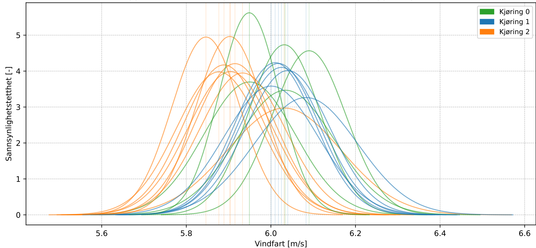
Approksimert fordeling av vindfart per kjøring, vinkler opptil 7 grader
