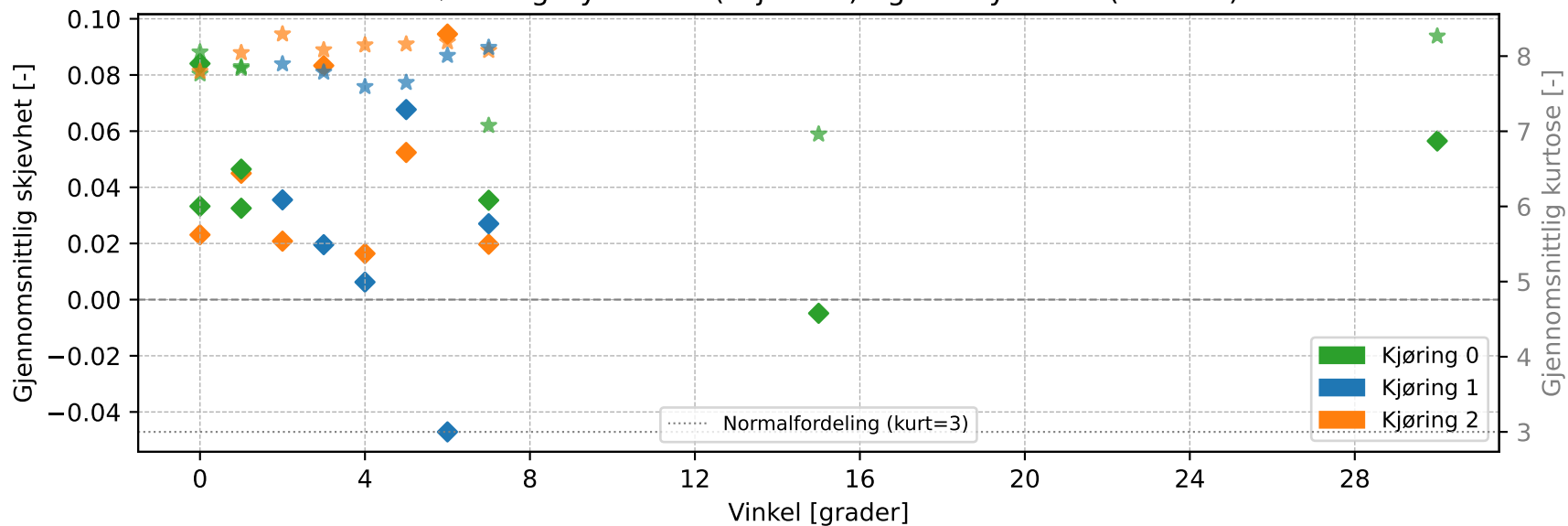
Strømningssymmetri (skjevhet) og haletykkelse (kurtose)
