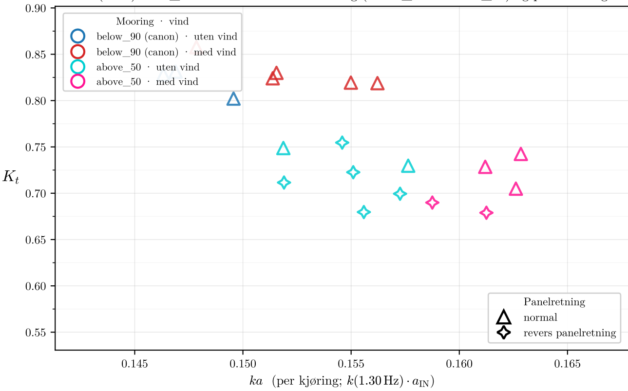
A3 (0.3V) — K_t vs ka ved 1.3 Hz · mooring (above_50 vs below_90) og panelretning
