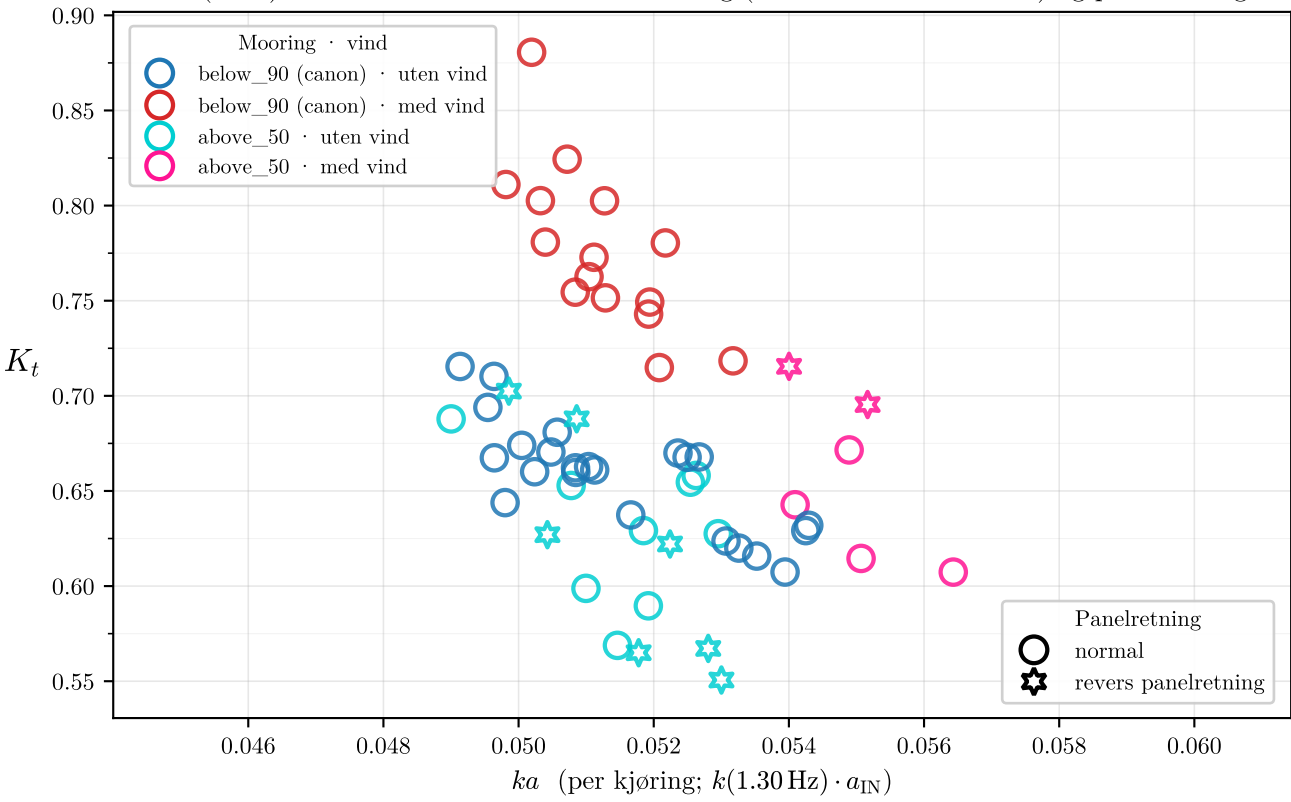
A1 (0.1V) — K_t vs ka ved 1.3 Hz · mooring (above_50 vs below_90) og panelretning
