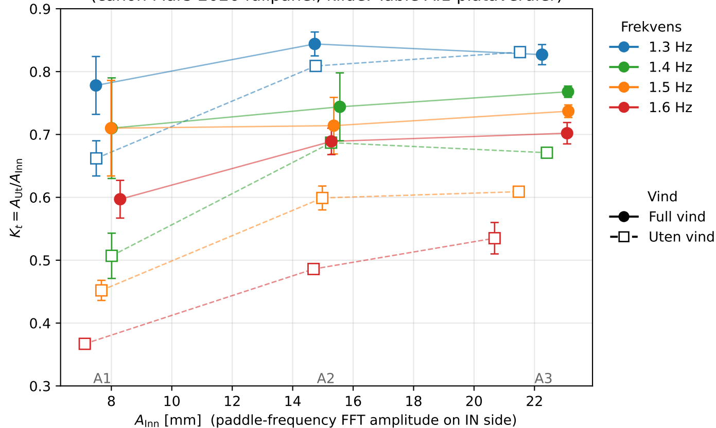
Transmisjonskoeffisient mot innkommende amplitude (canon Mars-2026 fullpanel, kilde: Table A.1 platåverdier)
