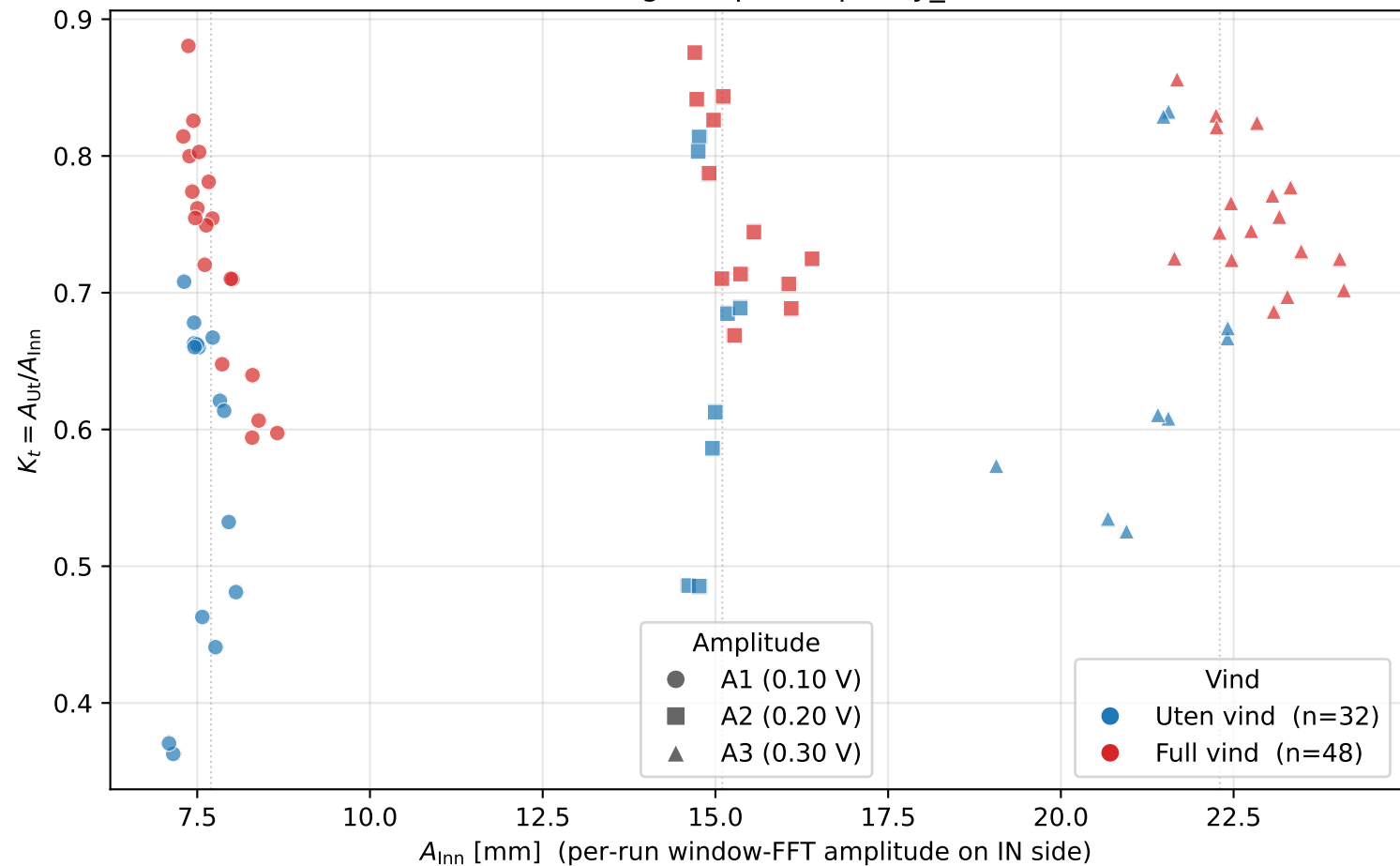
Transmisjonskoeffisient mot innkommende amplitude — alle målte canon-runs (March-2026 lowrange fullpanel quality_ok, N=80 runs)
