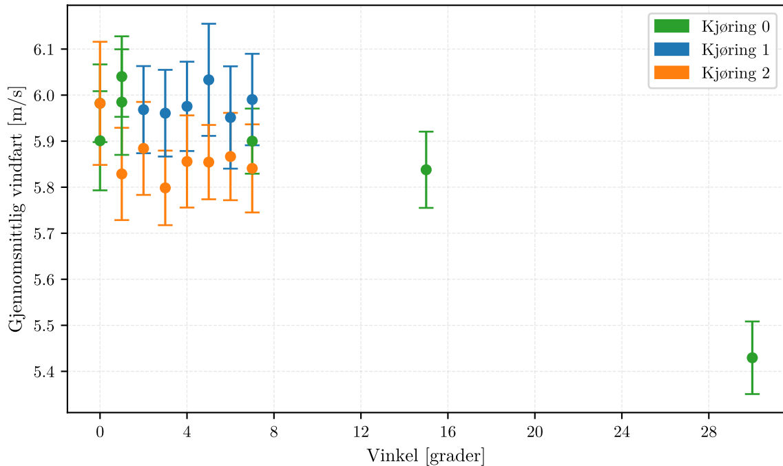
Estimert vindfart med samlet usikkerhet
