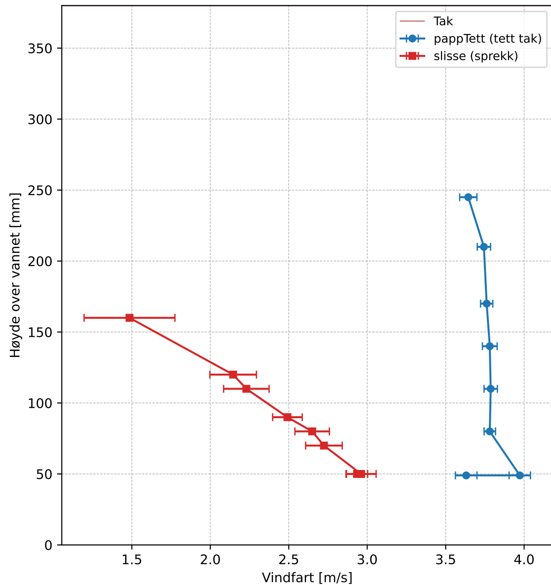
TunnelTest 7-tak — 07. november 2025, laveste vind pappTett (tett tak, gyldig) vs slisse (langsgående sprekk, annen fysikk)
