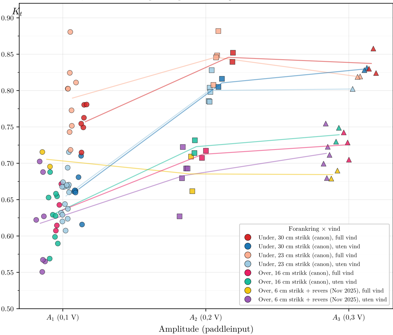
Tverrsnitt ved 1,3 Hz: K_t mot amplitude per forankring & vind
