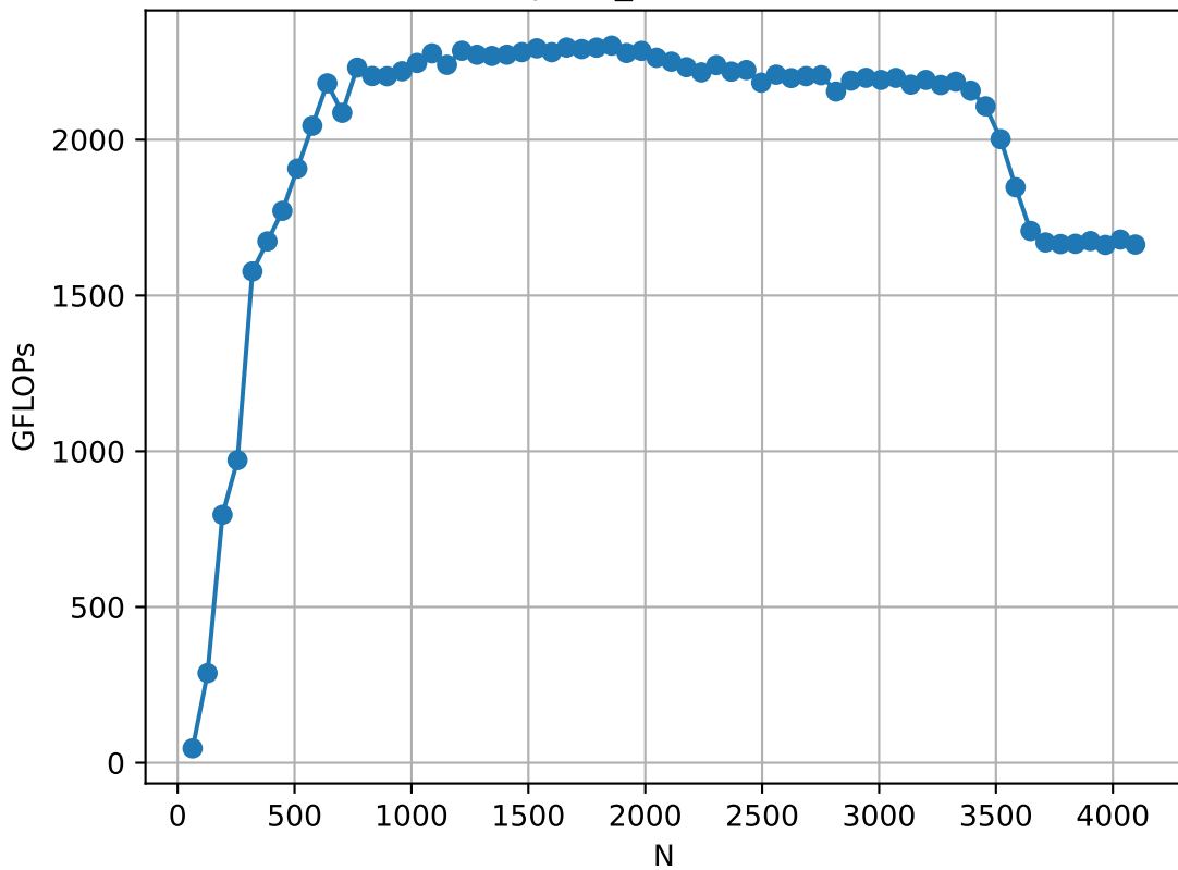
alpaka_full GFLOPs
