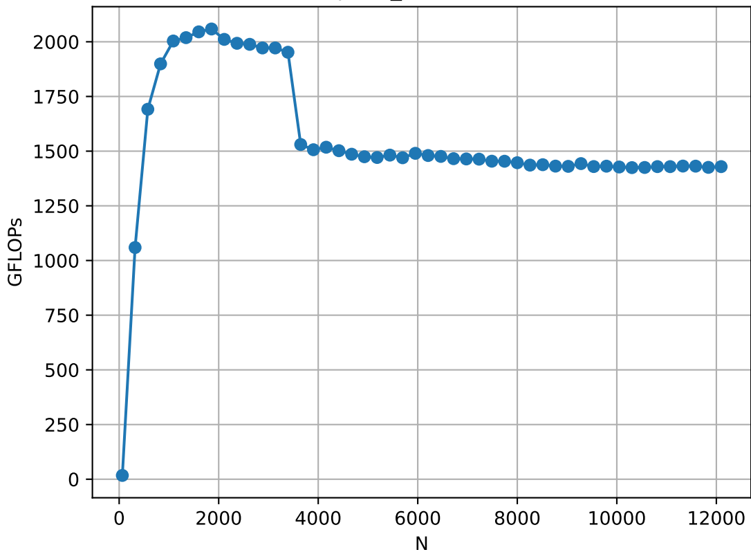
alpaka_full GFLOPs
