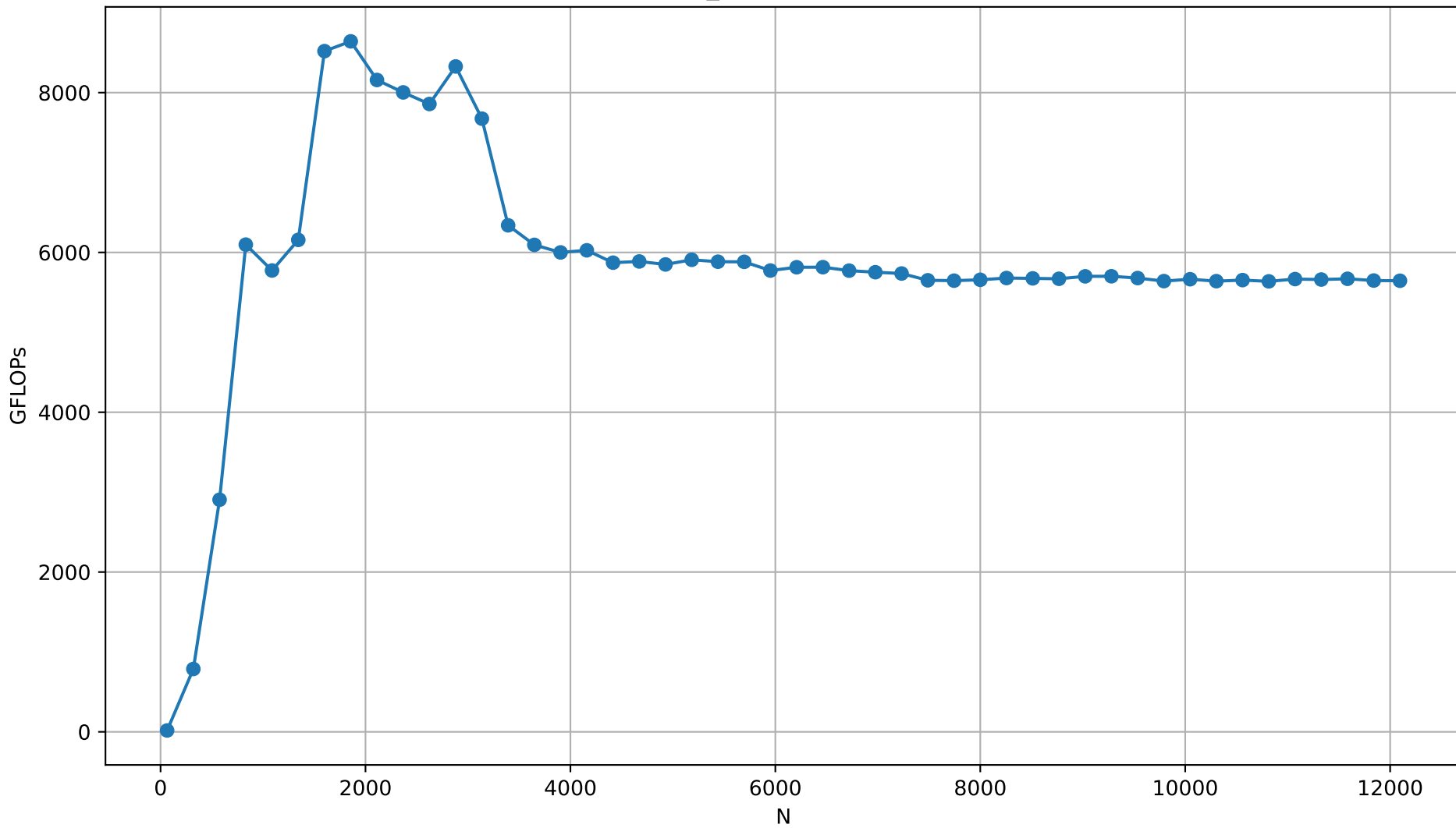
alpaka_full GFLOPs (float)
