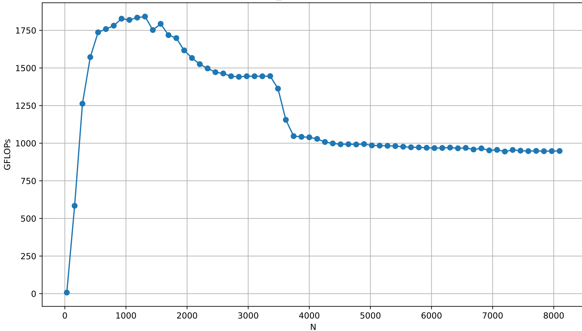
alpaka_naive GFLOPs (float)
