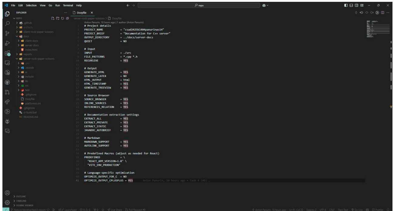
Рис.2. Doxyfile
