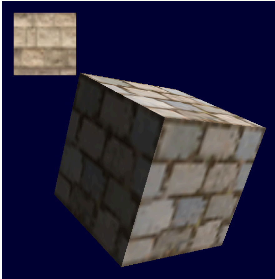
Figura 5: El motor en execució. El cub el genera el sistema de geometria amb una normal per cara; la textura i el color difús provenen d'un fitxer de material carregat des de disc. Les tres cares visibles reben il·luminacions diferents segons l'angle que formen amb la llum direccional: la dreta hi està encarada, la superior hi queda obliqua i l'esquerra n'està girada i només rep el terme ambient. El quadrilàter del cantó superior esquerre es dibuixa a la passada d'interfície, amb un material i una projecció diferents dels del món.
