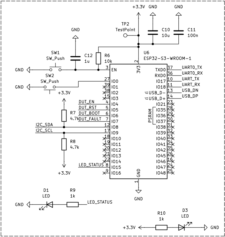
MCU ESP32-S3
