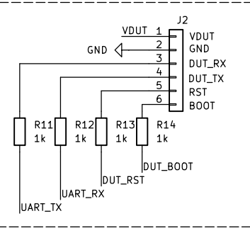
DUT connector
