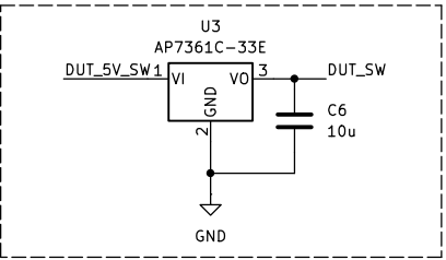
DUT 3.3 V regulator
