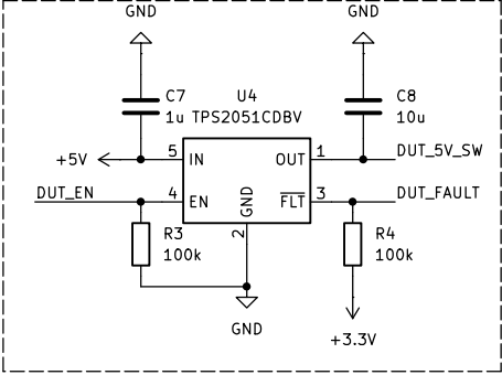
DUT power switch
