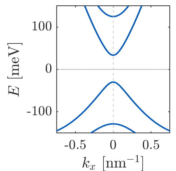
d) \text{MnBi}_2\text{Te}_4
