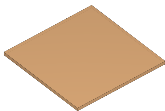
d) \text{MnBi}_2\text{Te}_4
