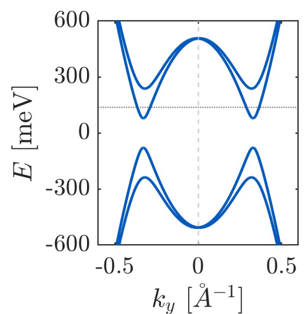
c) \text{WTe}_2
